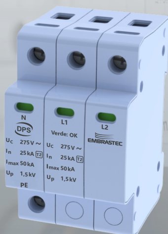
Trifásico
