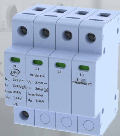
Trifásico+Neutro
