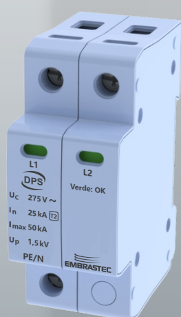
Bifásico
