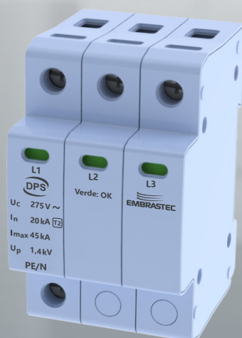
Bifásico+Neutro
